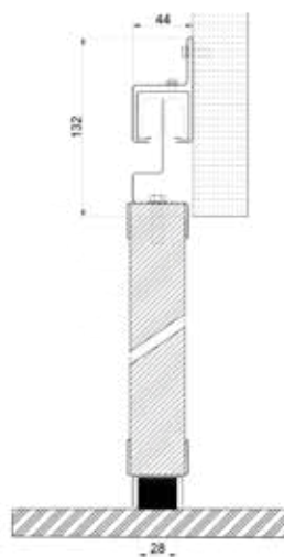
detail gegalvaniseerde rail
